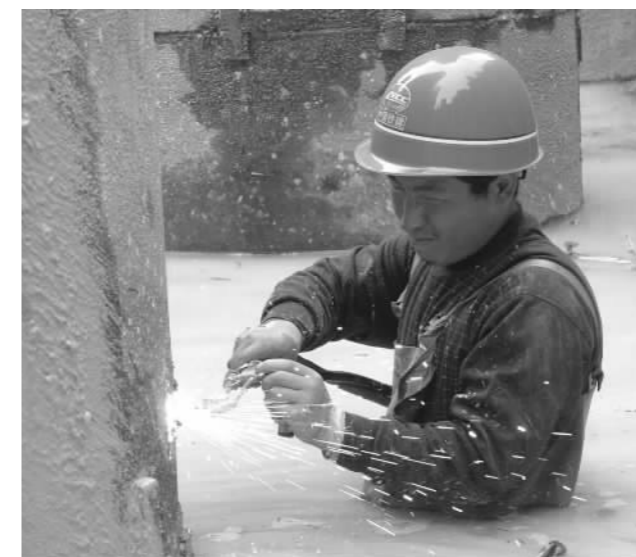
工人在齐腰深水中气割桥墩桩护筒。
