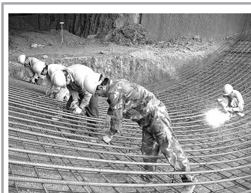
由十六局集团路桥公司参与施工的广(通)昆(明)铁路第3标段,自上场以来,项目部集中力量抓好征地拆迁和地方协调工作,在征地补偿无标准、征地工作困难的情况下,经过大家的共同努力,双洞村隧道率先开工,管段重点工程也陆续开工。图为施工人员正在进行隧道仰拱施工。黄洋洲 摄
